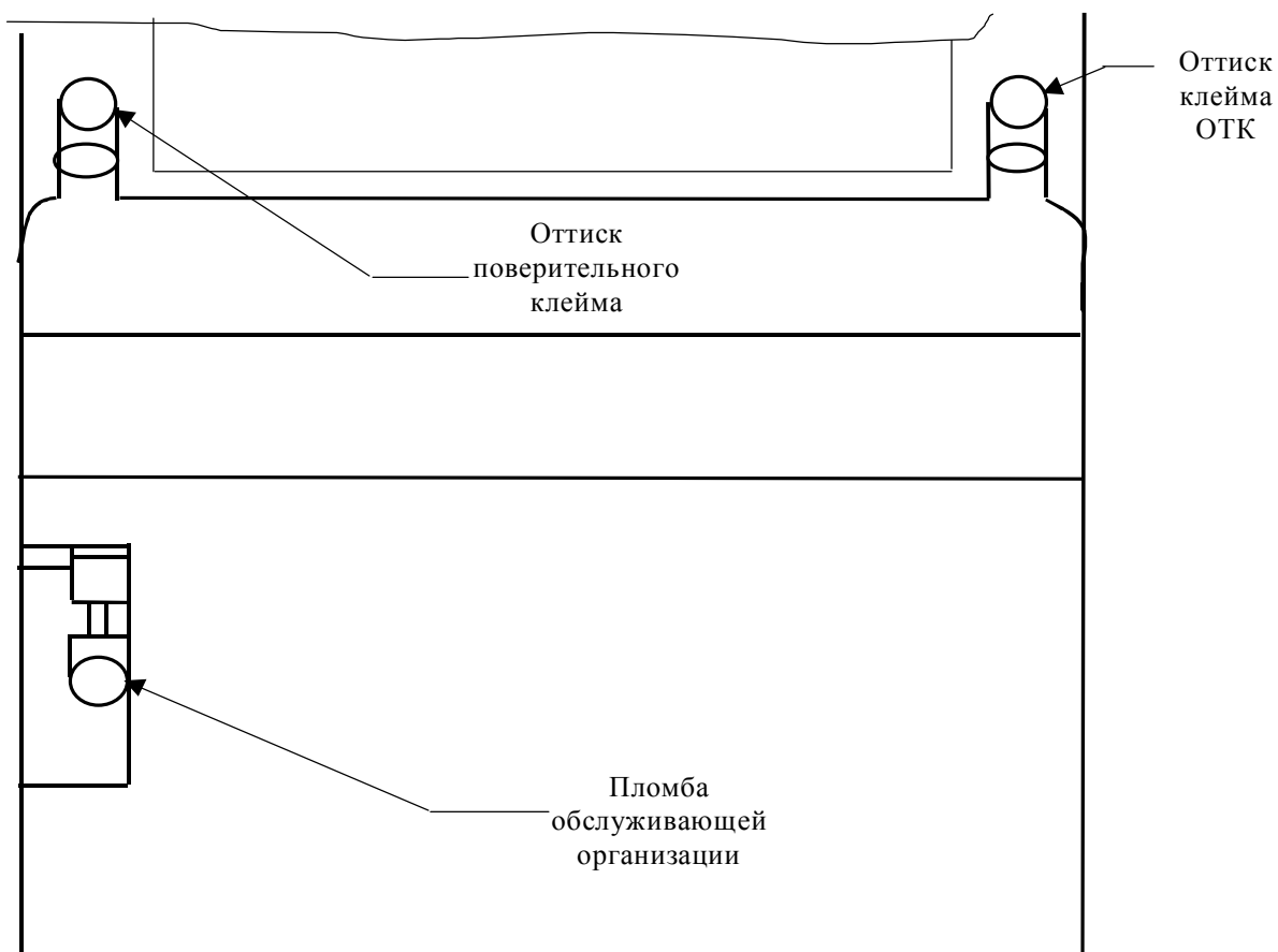
Рисунок 2 – Пломбирование счётчика
